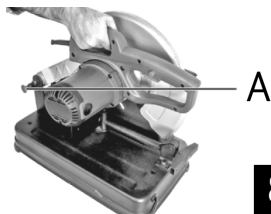
A - Rod switch
