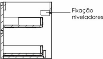
corte lateral
