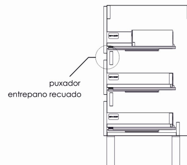
corte lateral
