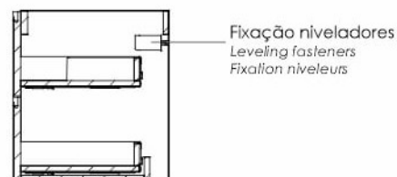
corde lateral section view | coupe latérale
